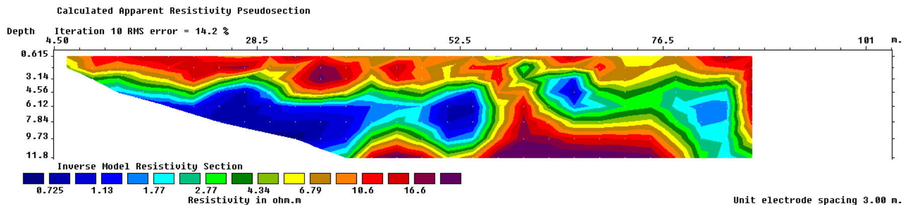
Figura 6. Inversión 2D de los datos de la matriz de resistividad a lo largo del perfil 1 que muestra la variación en la resistividad en el subsuelo, el color azul que representa la menor resistividad y el color rojo las zonas de mayor resistividad.
