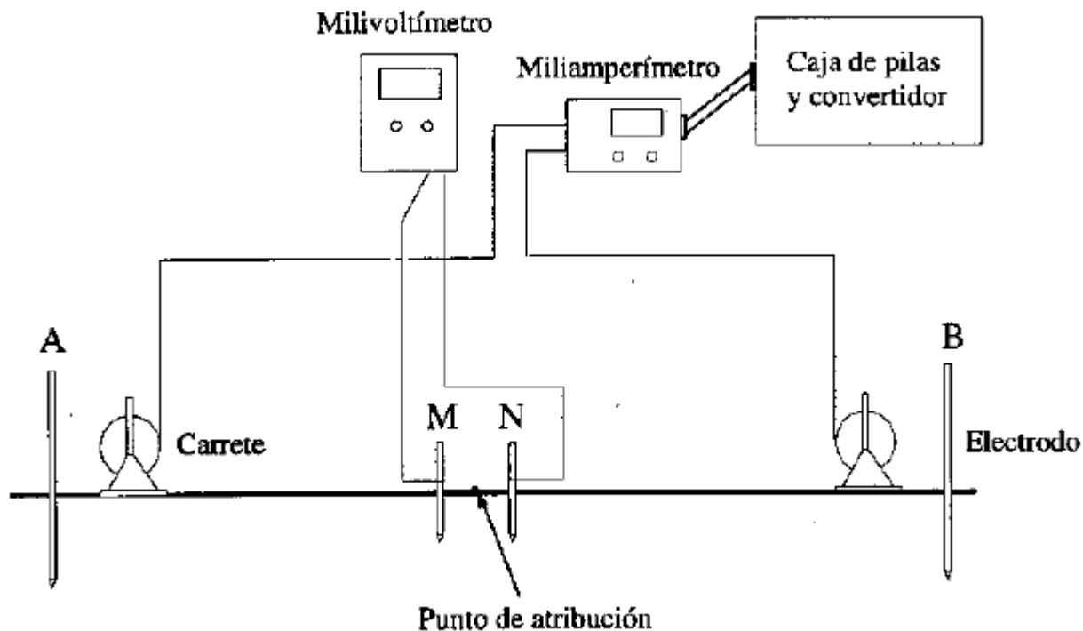
Figura 4. Esquema del tendido experimental de los sondeos eléctricos verticales utilizados.
