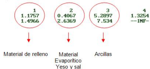
Figura 7. Sondeos eléctricos verticales en las ubicaciones SEV 1, SEV 5, y SEV 7, columna estratigráfica en los SEV 4 y SEV5.
