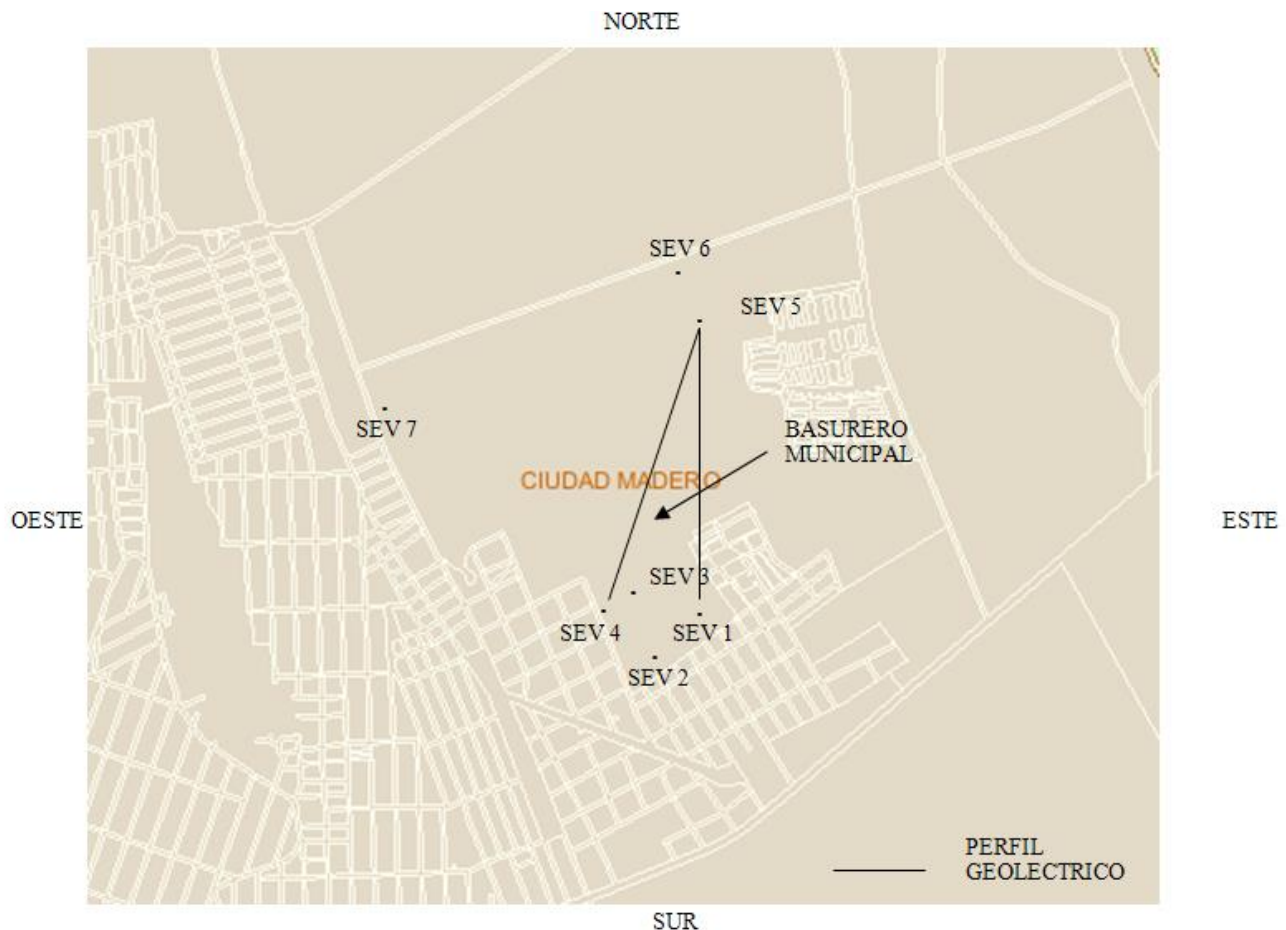
Figura 5. Esquema de ubicación del área de estudio y del tendido experimental de los sondeos eléctricos verticales realizados.
