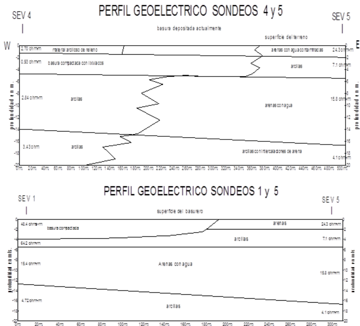
Figura 7. Perfil geoelectrico mostrando en la zona del vertedero municipal.
