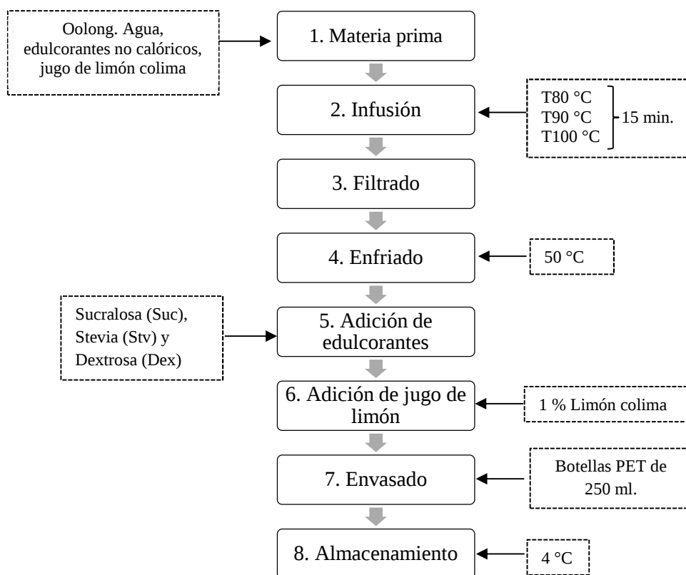
Figura 1. Diagrama de flujo del proceso de elaboración de una bebida a partir de una infusión de oolong adicionada con edulcorantes no calóricos
